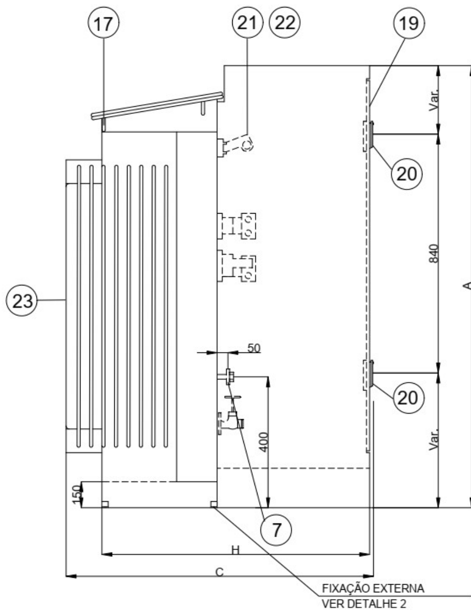
Figura 2 - Transformador pedestal radial – vista lateral
